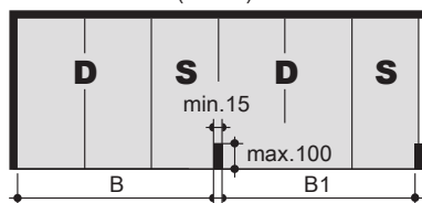
Unità combinate (6 auto)
